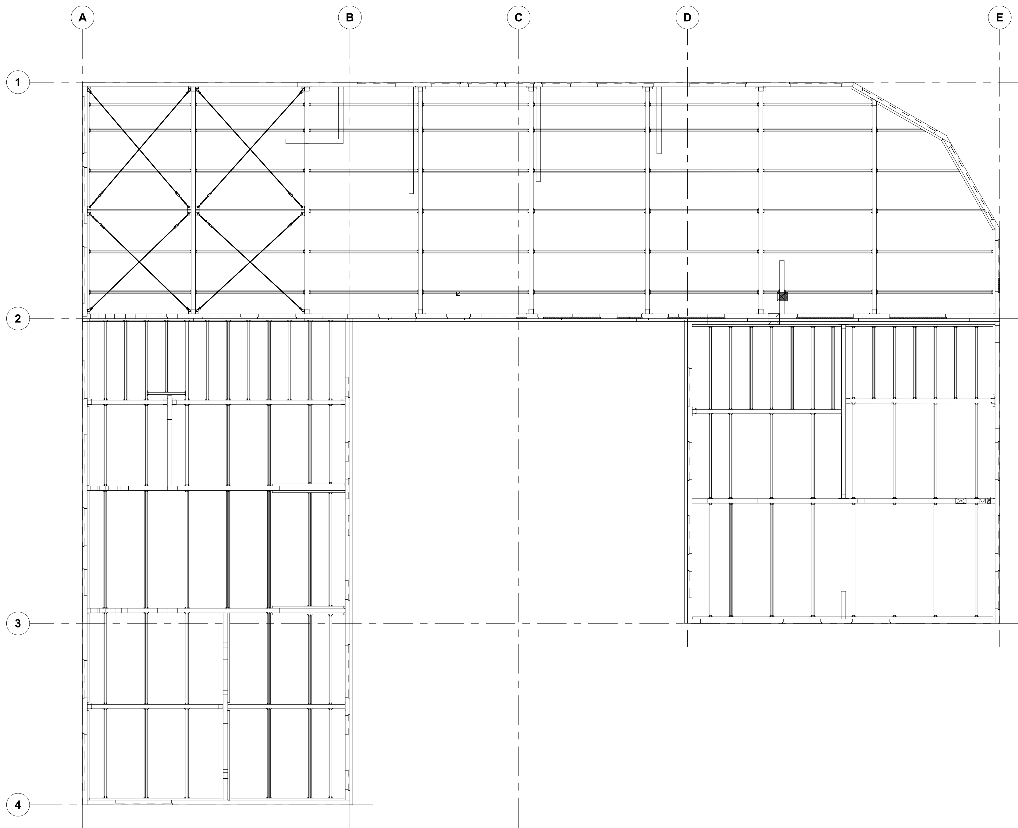
YFIRLITSMYND ÞAK 1 : 100
